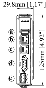
正视图
