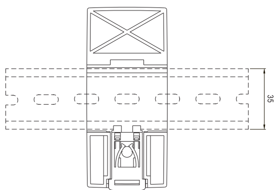
后视图
