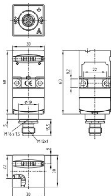
尺寸图（基本结构）
