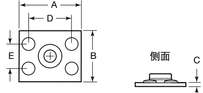
顶视图
