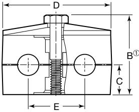
双支撑成套件
