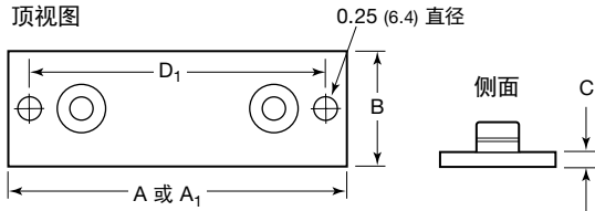
顶视图
