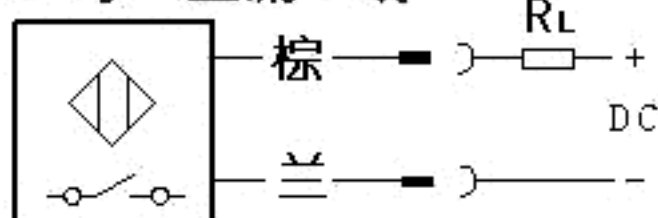
5号: 直流二线
