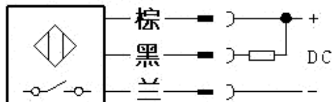
1号: NPN型
