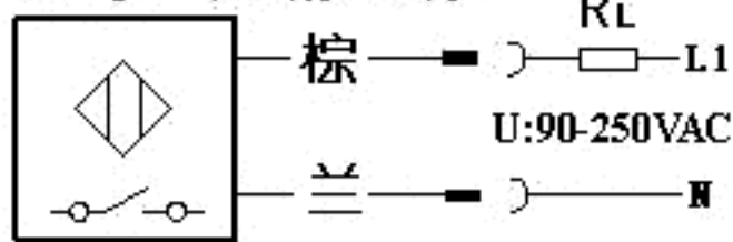
6号: 交流二线
