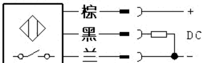
2号: PNP型
