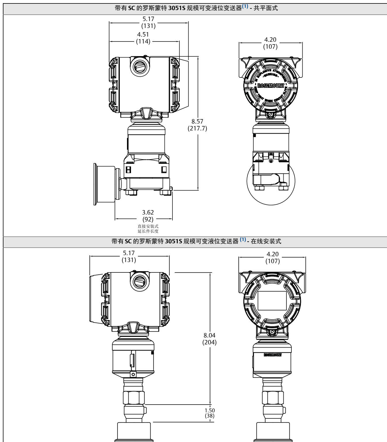
图 18. 带有 SC 密封件的罗斯蒙特 3051S 规模可变液位变送器
