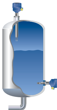
泵控制 / 限制检测
