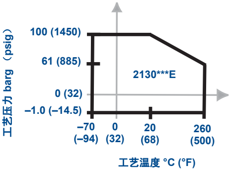
图 1. 工艺压力
