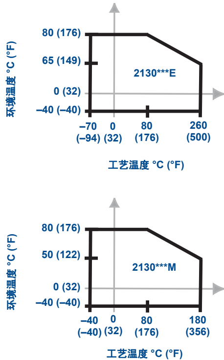
图 2. 工作温度
