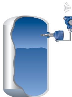
采用罗斯蒙特 702 型无线离散变送器的无线应用
