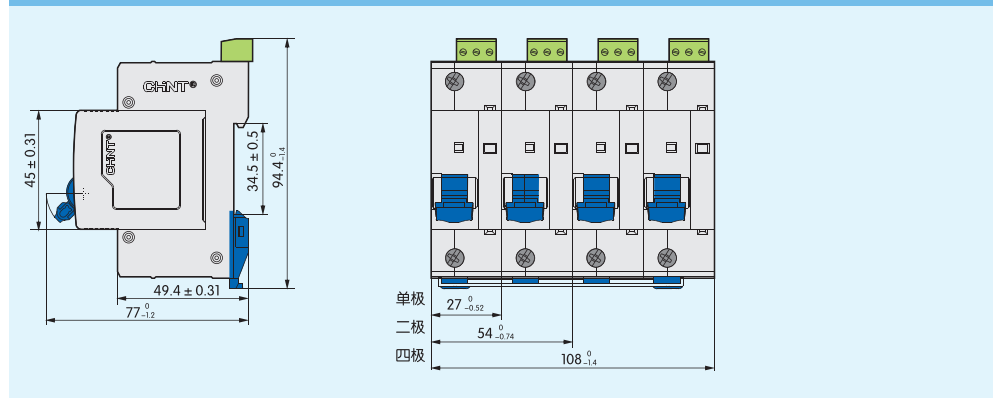
图1 NU210-40带远程信号输出接点电涌保护器外形及安装尺寸
