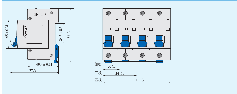
图2 NU210-40不带远程信号输出接点电涌保护器外形及安装尺寸
