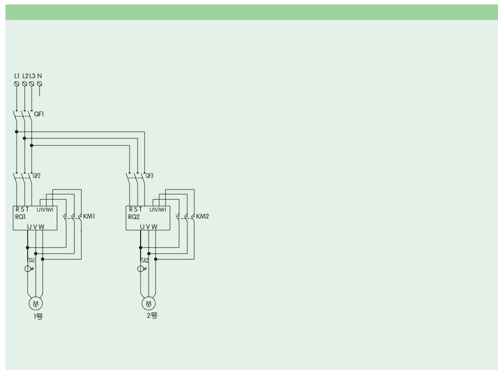
4.1 一用一备主电路图
