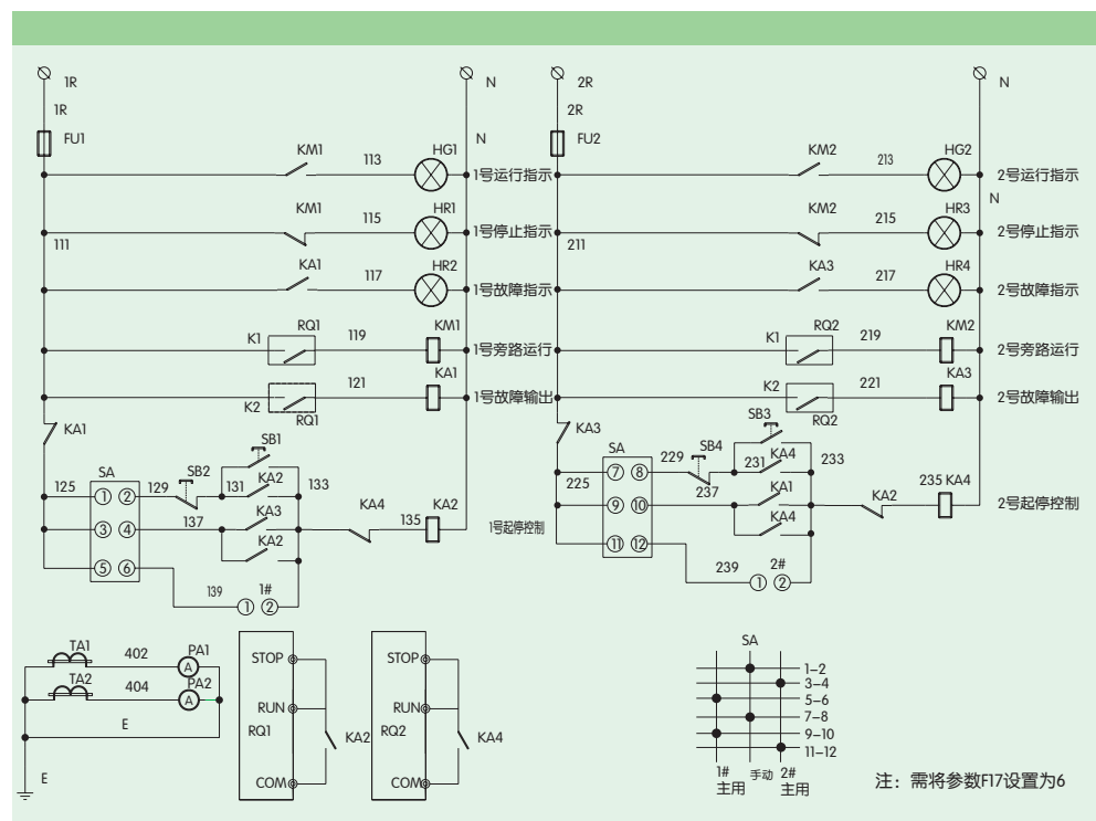
4.2 一用一备控制电路图
