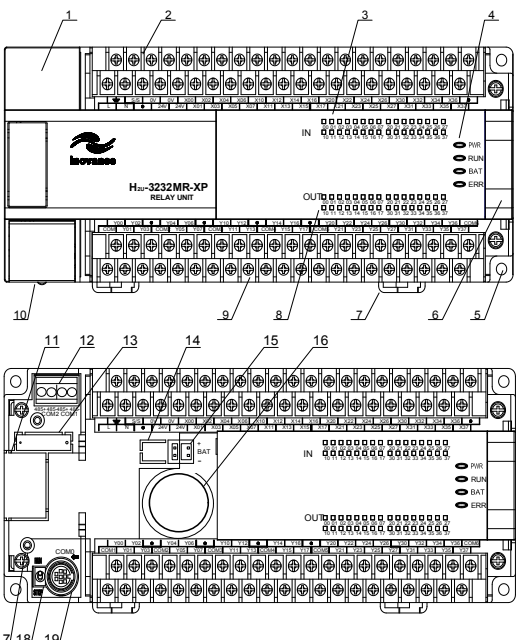
图 2 产品构造图
