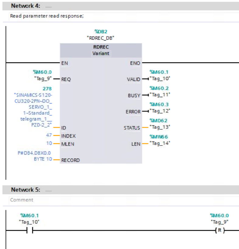
图 3-5 接收“读参数”请求的响应
