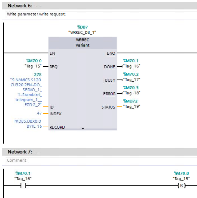
图 3-7 发送“写参数”请求
