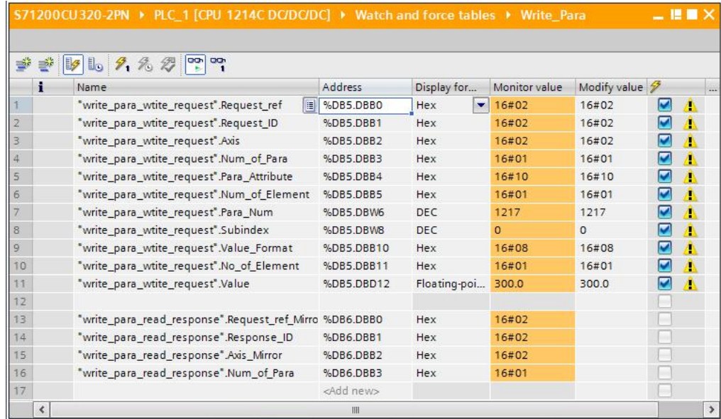
图 3-9 通过变量监控表写驱动参数
